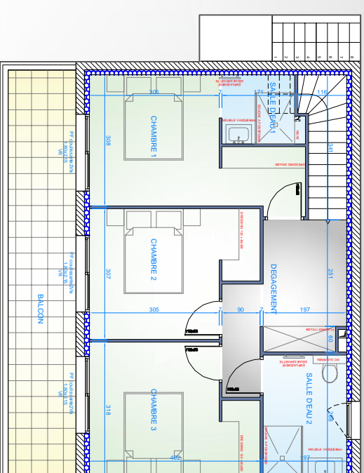
NIVEAU 2 - COIN NUIT
