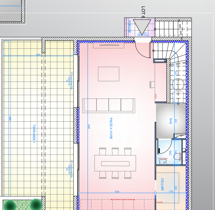
NIVEAU 1 - COIN JOUR
