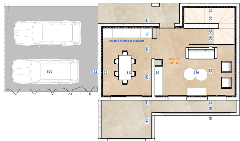
PLAN DU REZ-DE-CHAUSSEE
